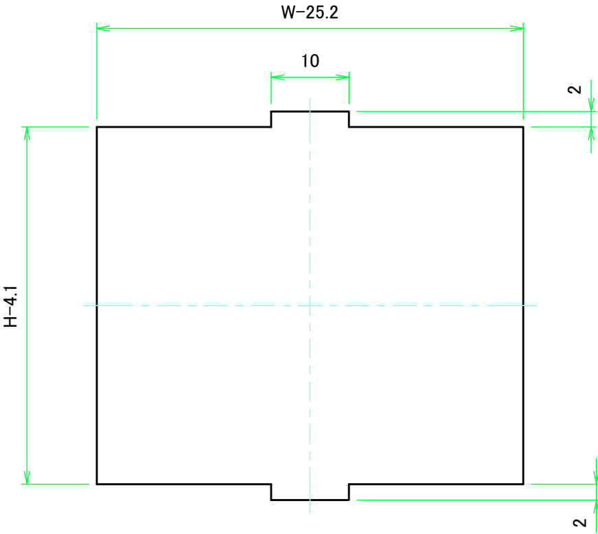
Wパネル1表面 / W Panel 1 Frontside
